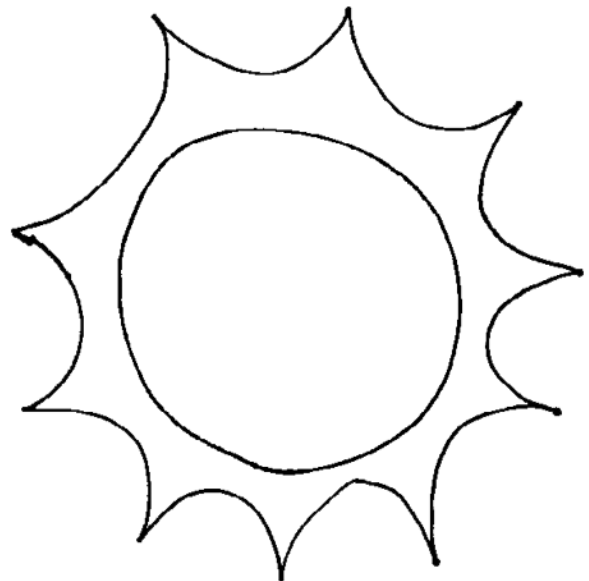
Sun
